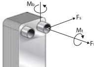
Figura 3. Cargas de conexión.
